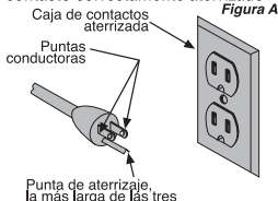
Punta de aterrizaje, la más larga de las tres
