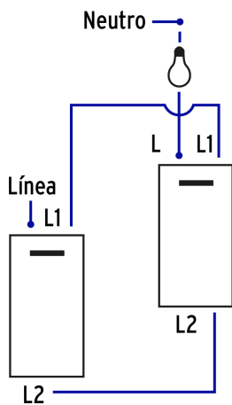
Interruptor 3 vías
