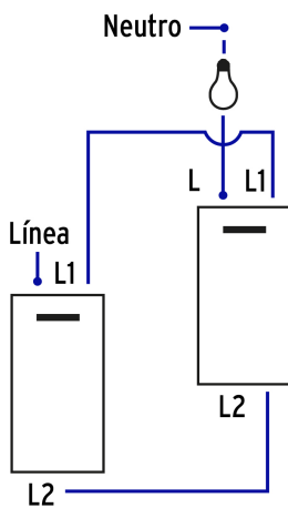
Interruptor 3 vías
