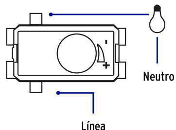
Diagrama de conexión
