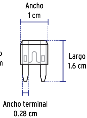
Fusible mini
