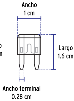
Fusible mini
