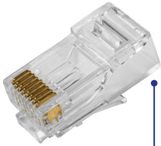
Cuerpo de policarbonato
