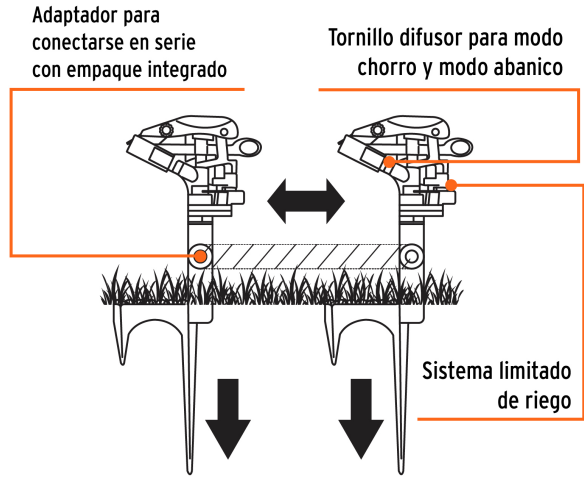
Gran alcance de riego al conectar 2 o más aspersores en serie
