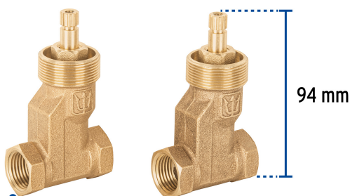
Conexión roscable de 1/2"-14 NPT
